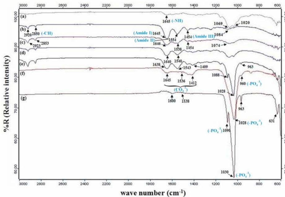
Fig. 1 ATR-FTIR spectra of (a) Chitosan (b) Gelatin (c) CS/GEL (d) CS/GEL/FHAP (e) CS/GEL/sFHAP (f) FHAP (g) sFHAP.
